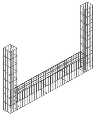
Podmurówka wraz ze słupami gabionowymi
